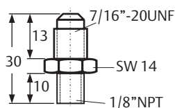
Адаптер 1/8" NPT внешняя резьба – 7/16"- 20UNF - внешняя резьба для установки непосредственно на компрессор № заказа: 800 316
