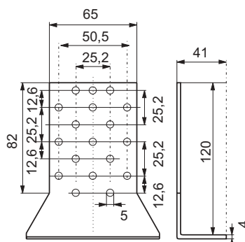
Универсальная монтажная пластина № заказа: 803 798
