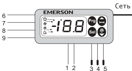
EC2-11x универсальный контроллер
