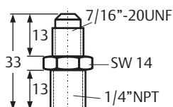
Адаптер 1/4 " NPT внешняя резьба – 7/16"- 20UNF - внешняя резьба для установки непосредственно на компрессор № заказа: 800 315
