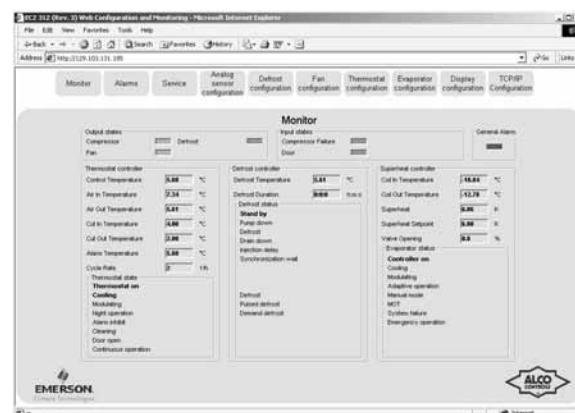
Пример просмотра интернет-страницы контроллера.
