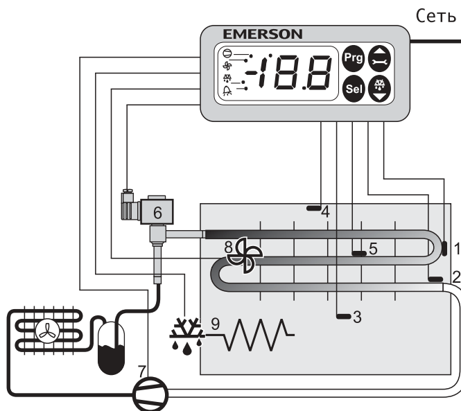
EC2-31x контроллер торгового оборудования (EXV, температура/температура)
