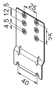
Монтажная скоба для приборов с крышкой Номер заказа: 803 801
