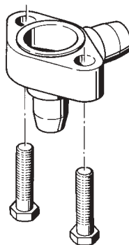
Угловой корпус
