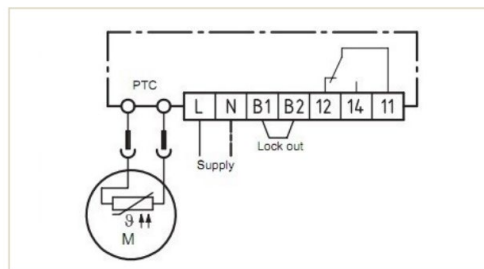
Схема подключения
