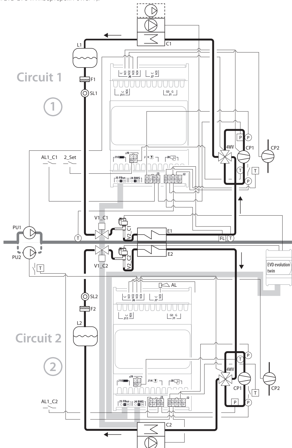
Поз. Описание Поз. Описание Поз. Описание C1/C2 Конденсатор 1/2 AL Тревога 4WV Реверсивный клапан E1/E2 Испаритель 1/2 F1/2 Фильтр-осушитель 1/2 P Датчик давления/реле давления V1_C1 Электромагнитный вентиль на контуре 1 FL Реле расхода T Датчик температуры/термостат V1_C2 Электромагнитный вентиль на контуре 2 CP1/2 Компрессор 1/2 SL1/2 Смотровое окошко жидкости 1/2 V2_C1 ЭРВ на контуре 1 PU1/2 Насос потребителя 1/2 AL1_ Внешний сигнал тревоги по контуру 1/2 V2_C2 ЭРВ на контуре 2 L1/2 Приемник жидкости 1/2 C1/2 2-я уставка
