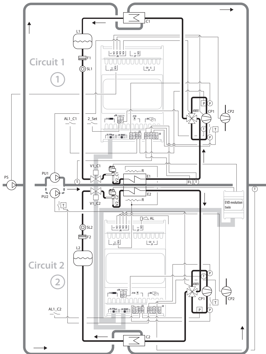
Поз. Описание Поз. Описание Поз. Описание C1/C2 Конденсатор 1/2 AL Тревога 4WV Ревверсивный клапан E1/E2 Испаритель 1/2 F1/2 Фильтр-осушитель 1/2 P Датчик давления/реле давления V1_C1 Электромагнитный вентиль на контуре 1 FL Реле расхода T Датчик температуры/термостат V1_C2 Электромагнитный вентиль на контуре 2 CP1/2 Компрессор 1/2 SL1/2 Смотровое окошко жидкости 1/2 V2_C1 ЭРВ на контуре 1 PU1/2 Насос потребителя 1/2 AL1_C1/2 Внешний сигнал тревоги по контуру 1/2 V2_C2 ЭРВ на контуре 2 L1/2 Приемник жидкости 1/2 R1/2 Нагреватель защиты от обмерзания R1/2 Frost protection heater PS Насос источника 2_Set 2-я уставка
