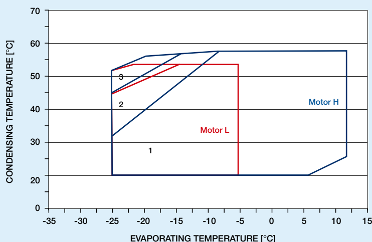
R407C APPLICATION LIMITS / LIMITI DI APPLICAZIONE R407C
