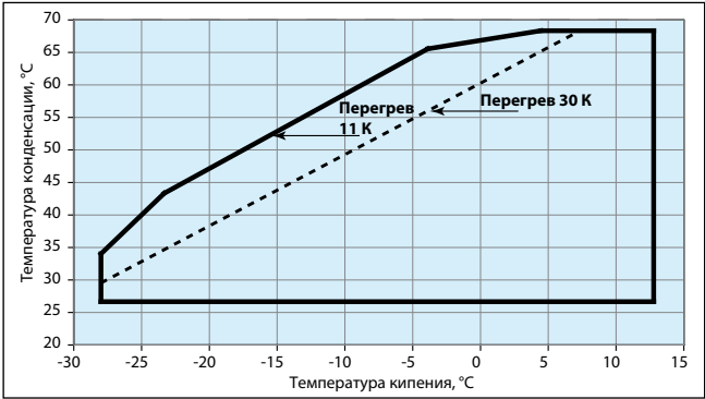
Область эксплуатации компрессоров Performer серии H с хладагентом R410A, тип T
