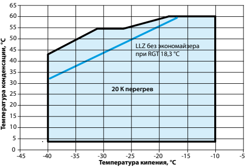
Диапазон работы низкотемпературной холодильной системы без экономайзера (R404A / R507)
