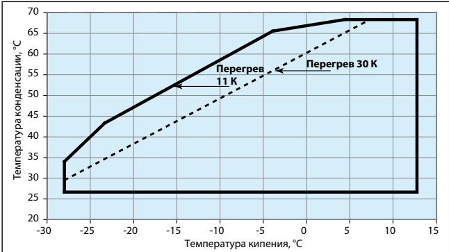
Область эксплуатации компрессоров Performer серии H с хладагентом R22
