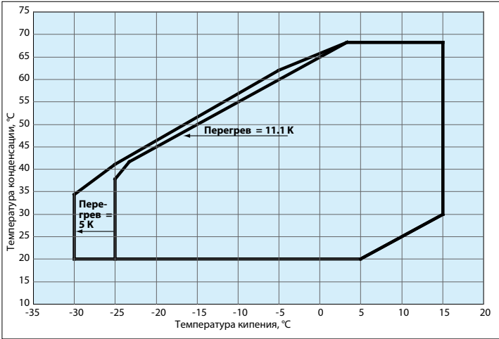
Область эксплуатации компрессоров Performer серии S с хладагентом R410A
