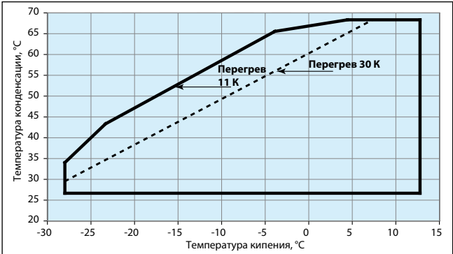
Область эксплуатации компрессоров Performer серии Н с хладагентом R407c
