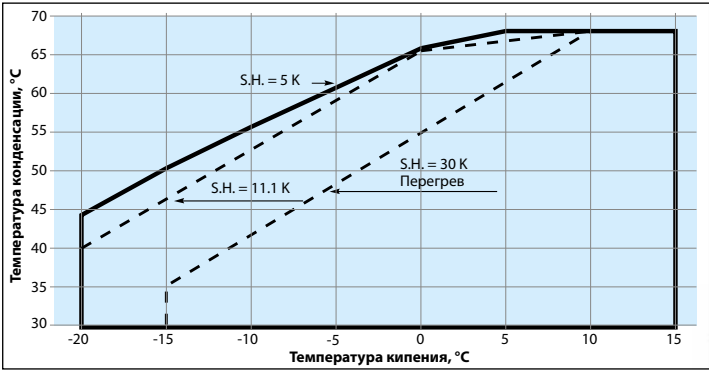
Область эксплуатации компрессоров Performer серии S с хладагентом R22
