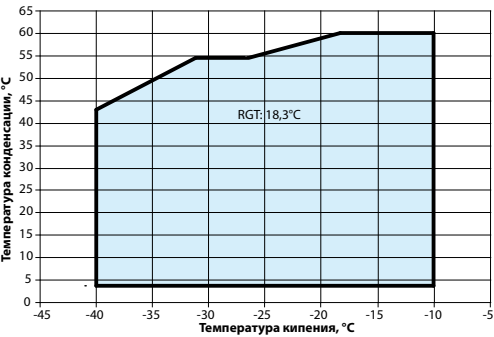
Диапазон работы низкотемпературной холодильной системы с экономайзером (R404A / R507)
