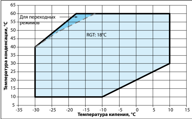
Область эксплуатации компрессоров серии MLZ с хладагентами R404A
