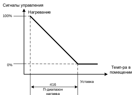
Управление нагревом при регулировании температуры
