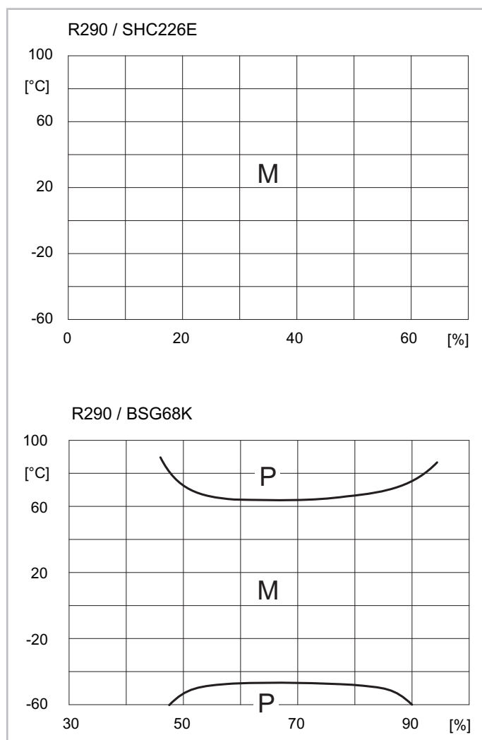
Рис. 8: Диаграммы смешиваемости для R290: Предельная температура зависит от содержания масла (% масла по массе в смеси хладагента с маслом).
