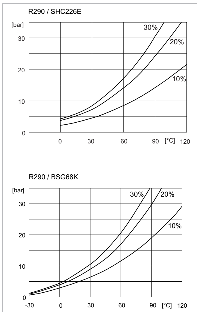
Рис. 9: Масла для R290: Давление хладагента в зависимости от температуры масла и содержания хладагента (% хладагента по массе в смеси масло-хладагент).
